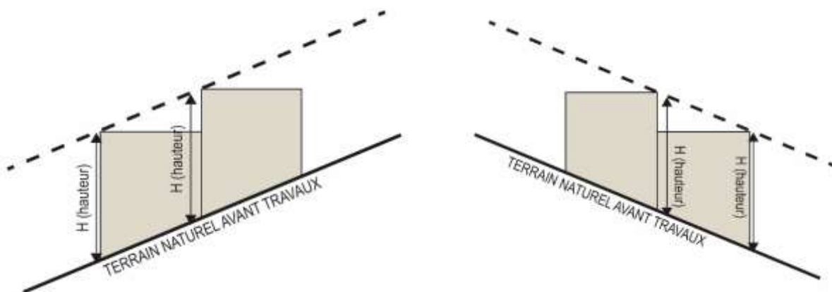
Schéma de mesure de la hauteur
